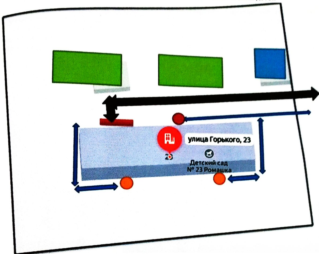
СХЕМА № 3. Организация дорожного движения в непосредственной близости от образовательного учреждения с размещением соответствующих технических средств организации дорожного движения, маршрутов движения детей
